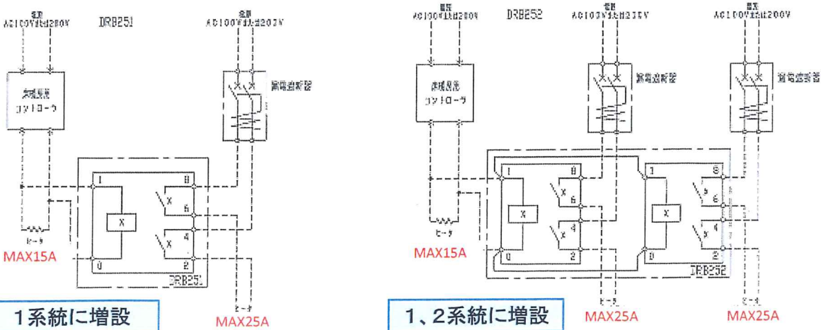
接続図(例)
