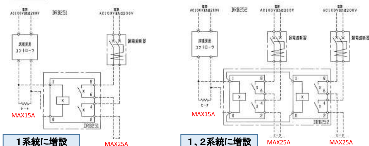
接続図(例)
